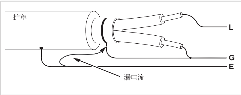
图 3.经改善的屏蔽端子连接
