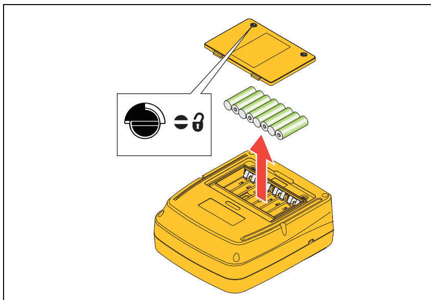
图 4. 更换电池
