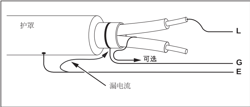
图 2.屏蔽端子连接
